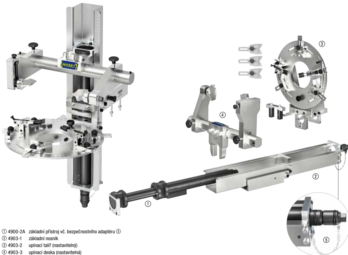
Stahovák pružin 4903/4
